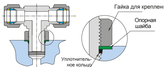
Окончательный монтаж регулируемого фитинга
